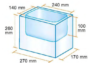
Mål på maskine og kar
